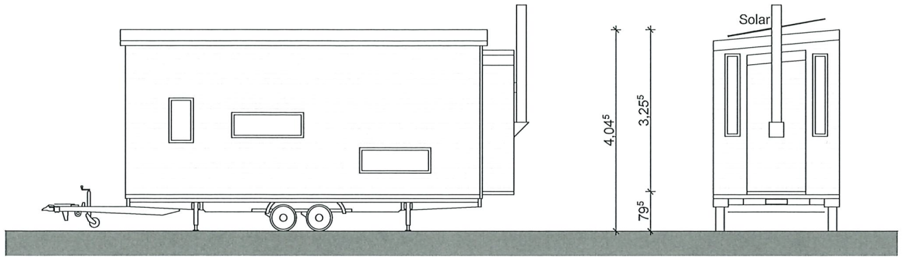
Ansicht SÜDEN
